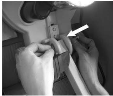
Stap 5 - Stel de bedieningshendel in en monteer de bevestigingschroef.
